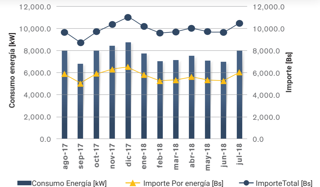
Figura 3: Consumo y costo anual del consumo de electricidad
