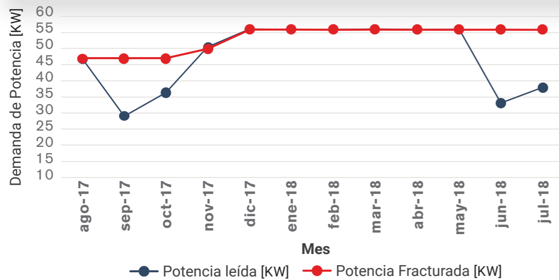
Figura 4: Demanda de potencia mensual leída y facturada
