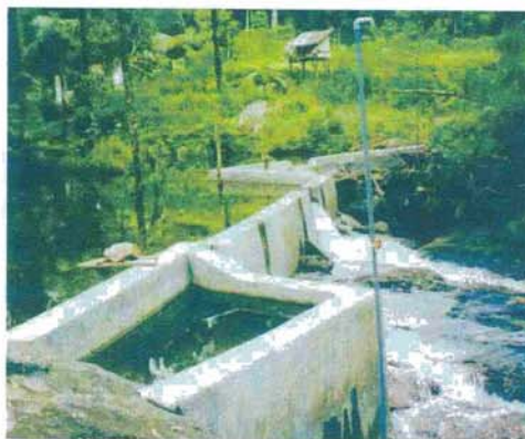
Foto 19 Pequena barragem com hidro- eléctrica de 14 kW
