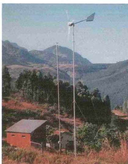
Foto 20 Turbina eólica de 1,2 kW em Manicaland, Zimbabwe
