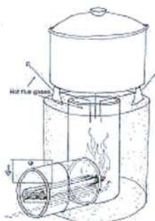
Foto 6 fogão tipo "foguete" para materiais combustíveis alternativos
