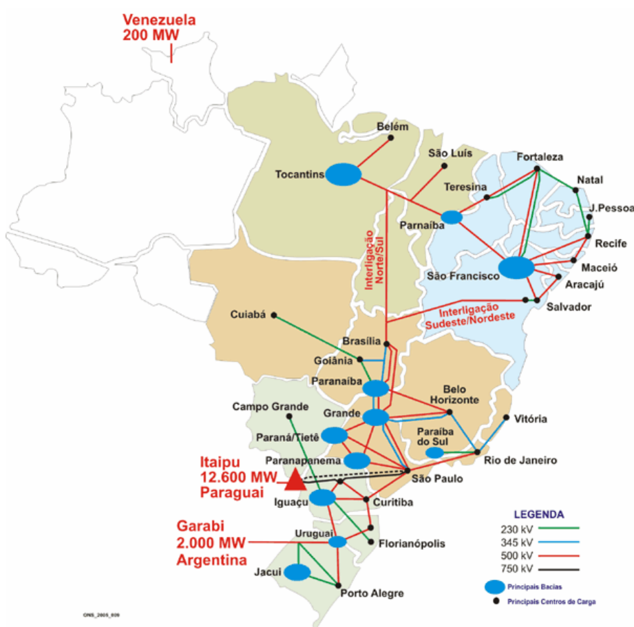
Figura 7 Sistema de Distribuição de Energia no Brasil, 2005 Fonte: ONS (2005)
