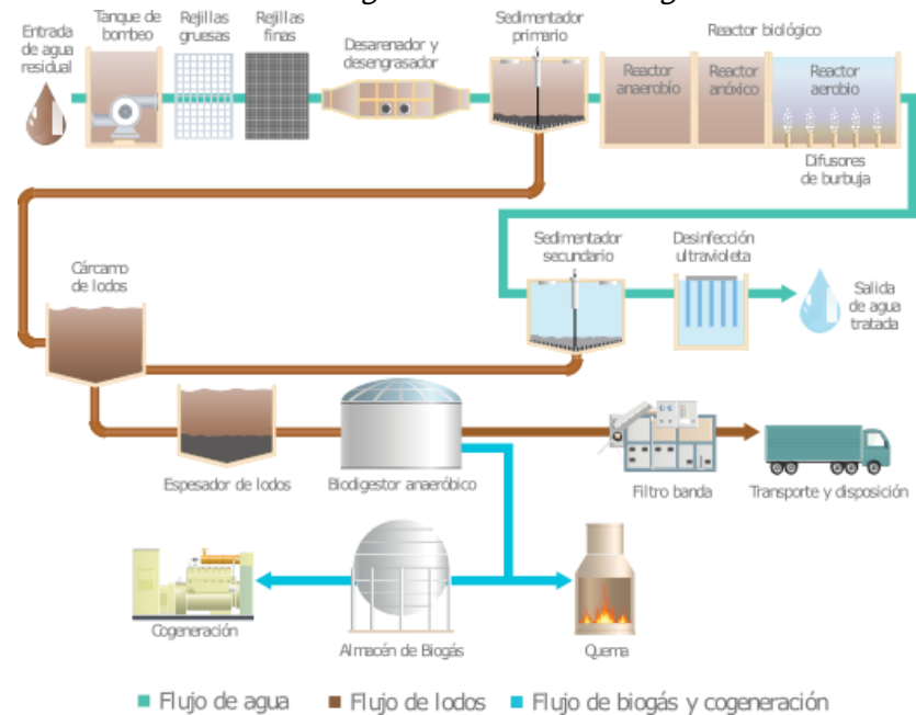
Figura 78. Aprovechamiento energético de biogás por tratamiento de lodos de planta de tratamiento “El Ahogado”. Fuente: (GIZ, 2018)
