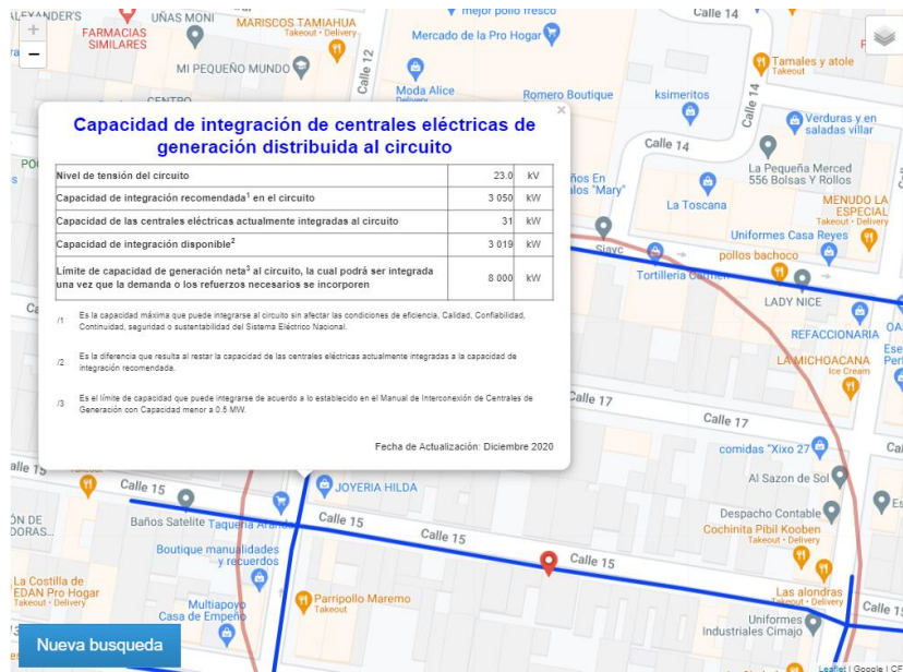
Figura 47. Capacidad de integración del circuito de la Calle 12 (Casi vertical) que aparenta ser distinto al de la Calle 19 (casi horizontal). Sin embargo, los datos son idénticos, mostrando que se trata del mismo circuito. Tomado de (CFE Distribución, 2018)
