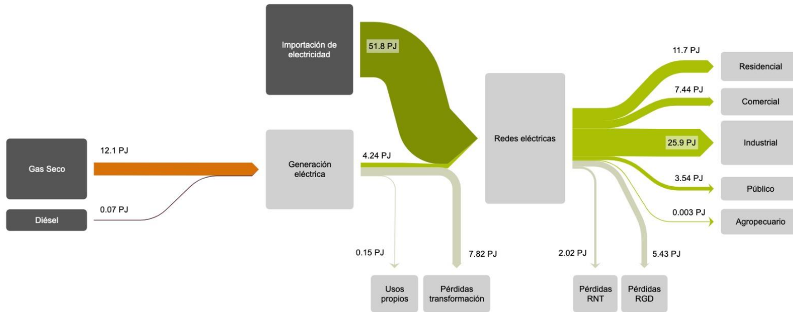
Figura 13 Diagrama de Sankey de la cadena energética de la electricidad en la Ciudad de México. Fuente: Elaboración propia con base en datos de: (CRE, 2020), (SENER, 2021) y (OBTREN, 2021)
