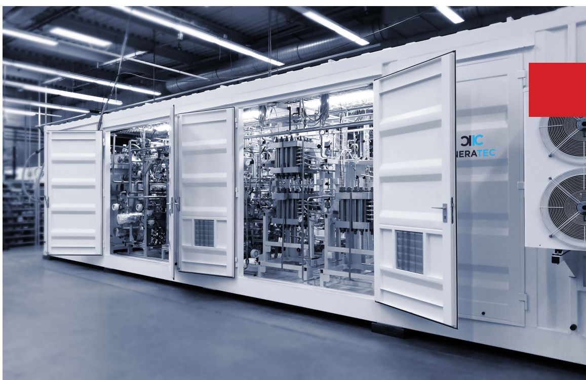
Planta Power-to-Liquid para la producción de e-fuels. © INERATEC
